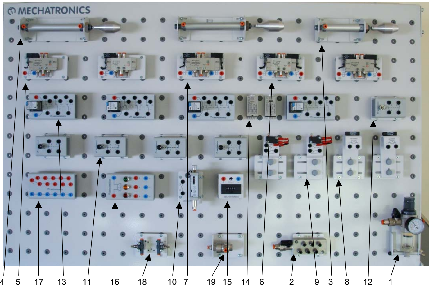
Stel componenten – Elektro-pneumatiek, niveau 1 (MEP2003) bevat eveneens de 24 V gelijkspanningsvoeding en een stel elektrische verbindingssnoeren die hierboven niet zijn afgebeeld.
