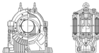
Doorsnede tekening hydrodynamisch lagerblok
