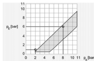
Diagram drukschakelaar
