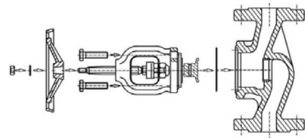
Montagetekening cilinderklep afsluiter
